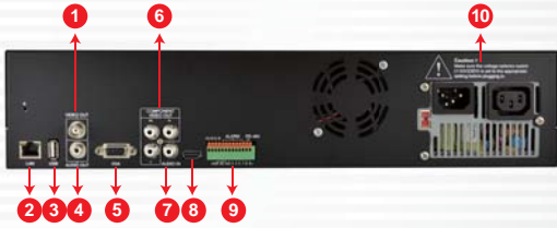
背板
